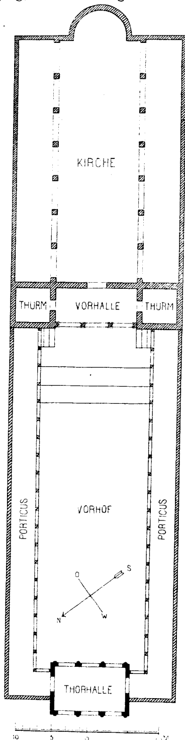
Nr. 1a. Grundriss der fränkischen Kirchenanlage.
