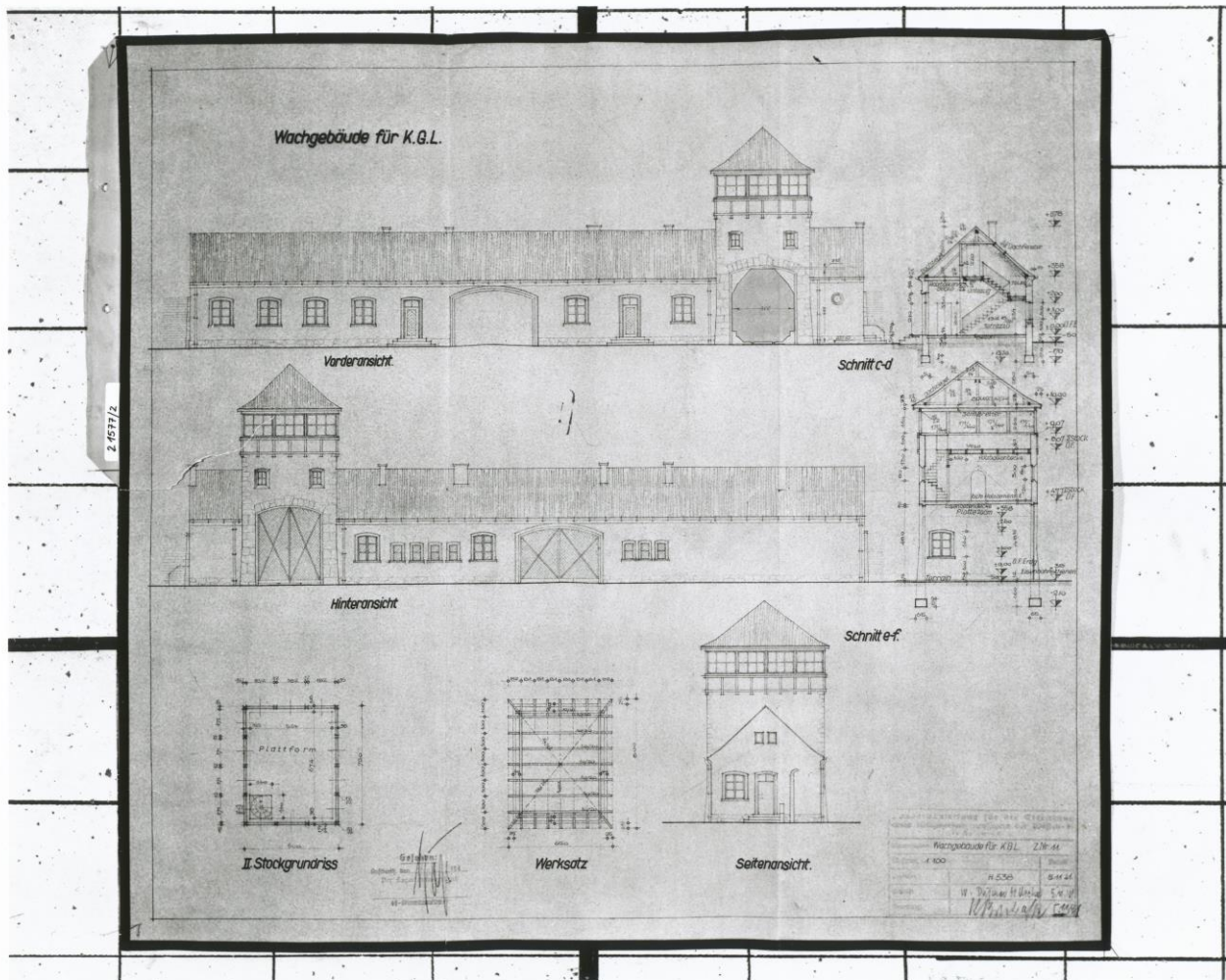
Wachgebäude für K.G.L., Plantransparent im Maßstab 1:100, 15.11.1941 vor der Erweiterung. Planrepro von Robert Jan van Pelt, University of Waterloo, School of Architecture, Canada.
