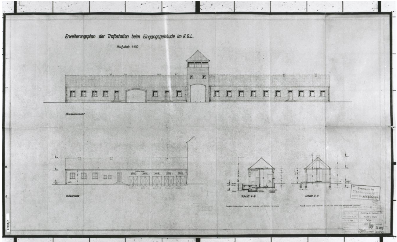
Erweiterungsplan, Plantransparent im Maßstab 1:100, 26.10.1943
