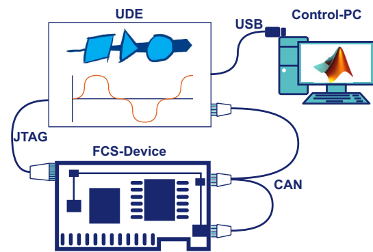
Fig. 6 Test setup
