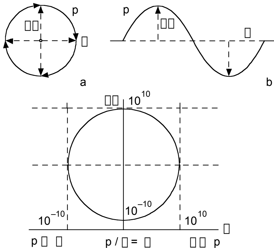
Abb. 5 Eine vergleichende Gegenüberstellung der Wellenformen. Sowohl sphärische Welle (a) als auch ausgedehnte Welle (b) können mit gleichen Zustandsgrößen beschrieben werden ( p , \lambda , \pi ). Ein Diagramm unten veranschaulicht die Verhältnisse zwischen diesen Zustandsgrößen.
