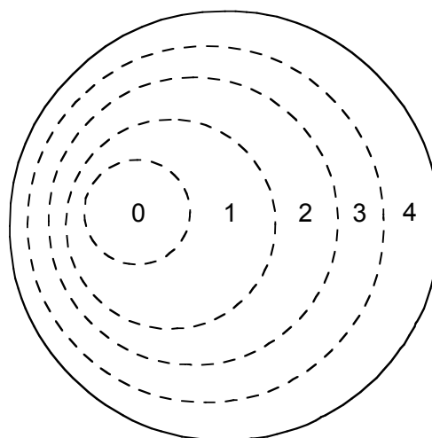
Abb. 9 Das Zustandsdiagramm des Raumes. Die Zahlen stehen für Vakuum (0), Plasma (1),
