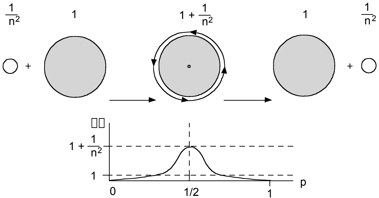
Abb. 7 Eine veralgemeinerte Darstellung der Periodizität. Während das Atom eine elementare Quantität aufnimmt (Absorption), dehnt es aus (Ausdehnung wenn n > 1 , Unterteilung wenn n = 1 ). Bei \lambda = 1 befindet sich Atom in einem gleichgewichtigen Zustand, während \lambda = 1 + 1/n^2 die angeregte Zustände sind. Die angeregte Zustände resultieren in einer Entspannung (Emission bzw. in Form einer Welle, die sich im Raum ausdehnt). Der Abstand zwischen Absorption und Emission bezeichnet man als die Schwingungsperiode p = 1 .
