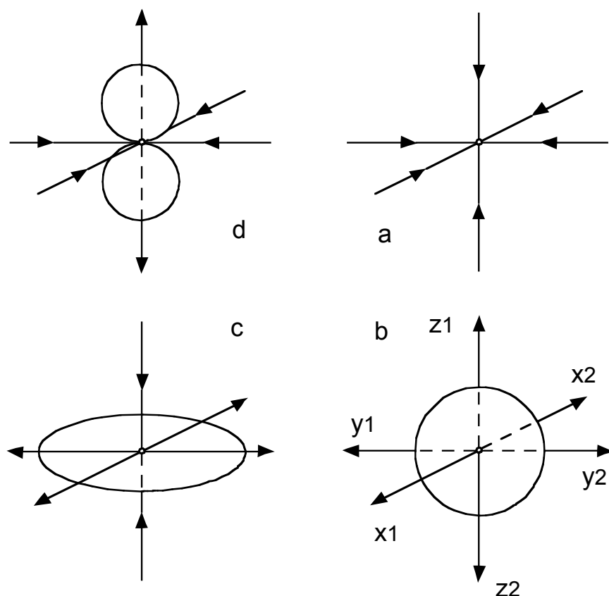
Abb. 4 Koordinatensysteme in einem multifocalen Universum. Jeder Punkt des Raumes stellt
