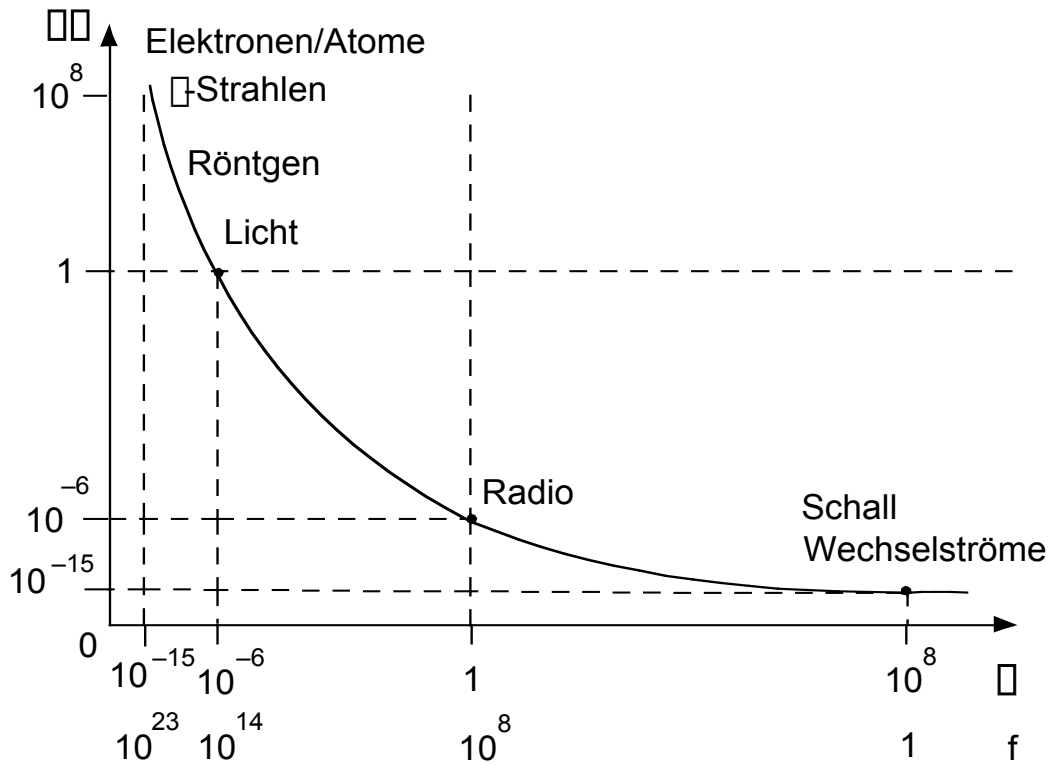
Abb. 8 Das geometrische Wellen-Spektrum. Die Verhältnisse zwischen den Wellenklassen sind in einem Diagramm zusammengefasst, und beziehen sich auf die Positionen, wo die Maßgrößen \lambda und f jeweils den Wert von 1 annehmen. Das Spektrum bekommt damit die Symmetrie-Achsen, die den Raum dieses Diagramm unterteilen, was bei einer traditionellen Darstellung nicht zum Vorschein kommt.
