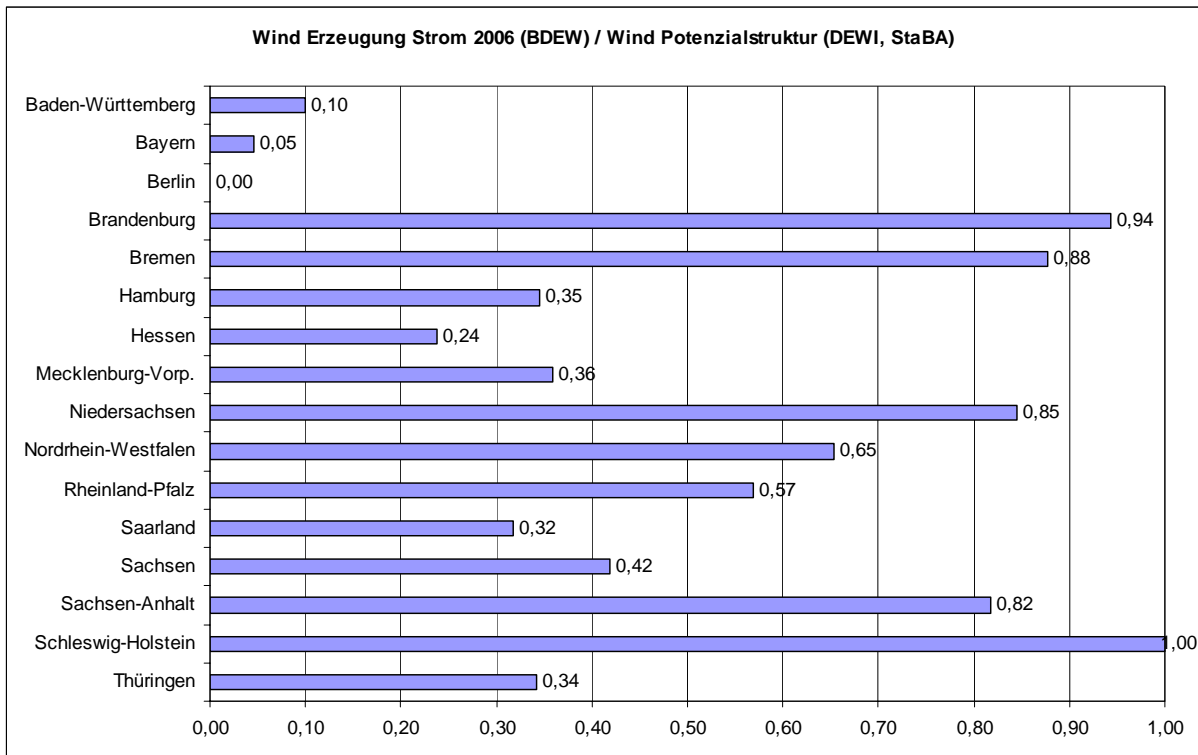
Abbildung 19: Indikator 2A-5: Windstromerzeugung 2006 bezogen auf das Vergleichspotenzial
